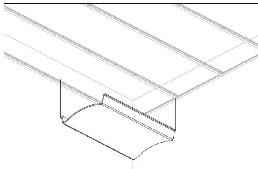
התקנת אריח ARCHI ע"ג קונס' T
