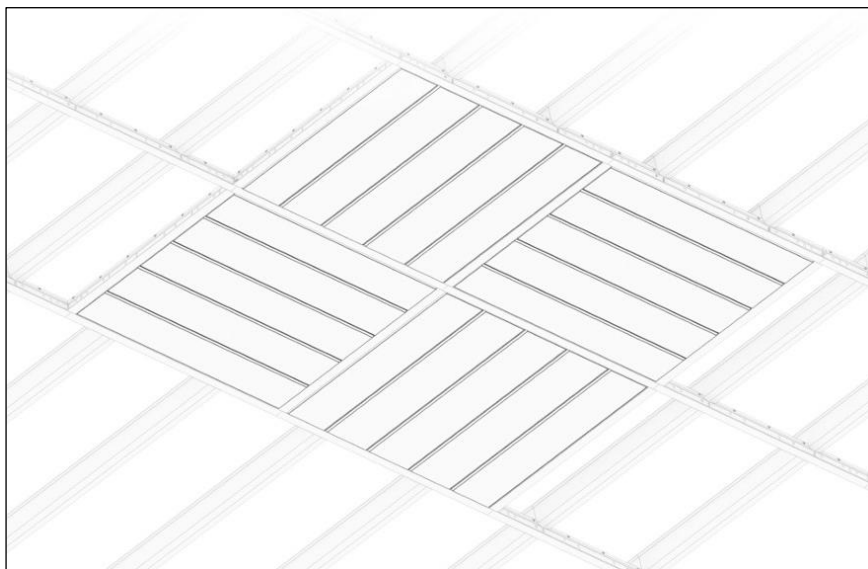
התקנת אריח MODULINE ע"ג קונסט' T
