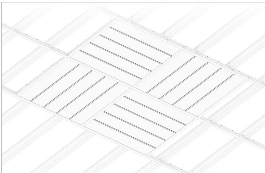
התקנת אריח MODULINE ע"ג קונס"ט
