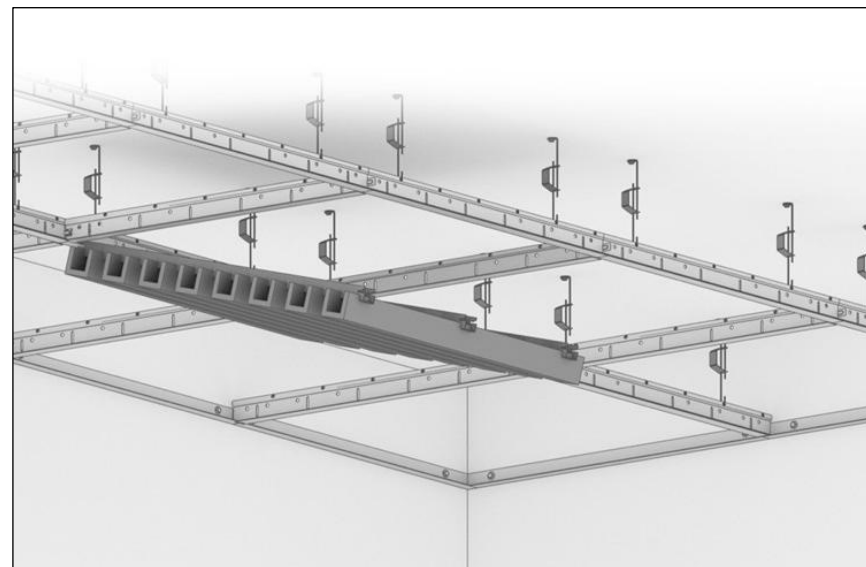
התקנת אריח FELT LINE ע"ג קונס' T
