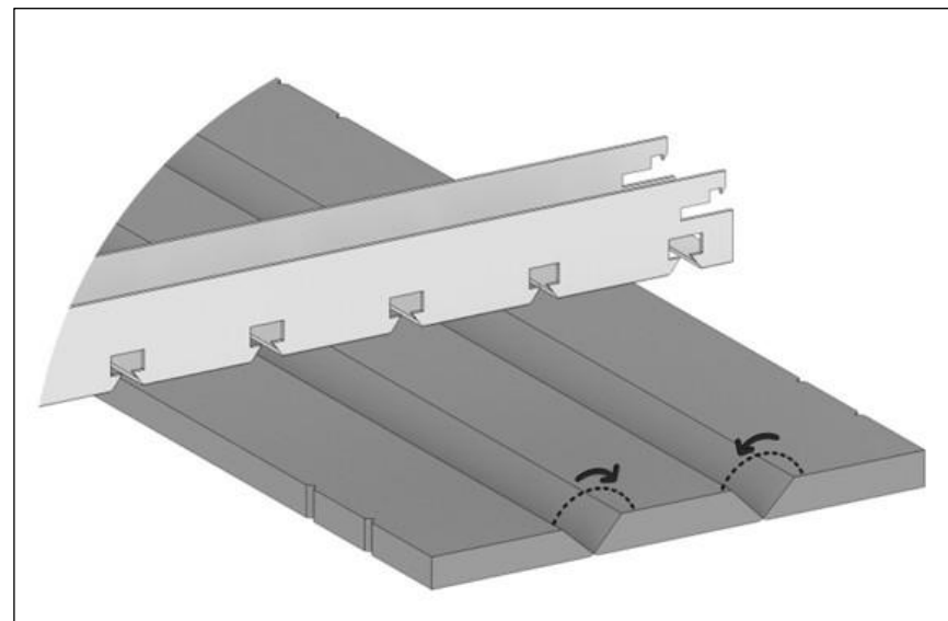
יש לקפל כל למלה לצורת U - 8 למלות לכל אריח
