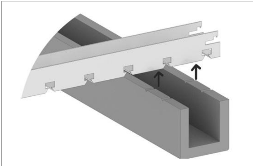
יש להכניס את הגשרים אל ה"שיניים" הייעודיות של כל למלה
