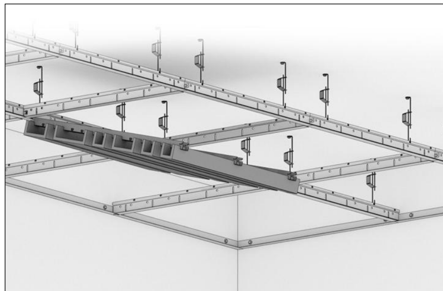
התקנת אריח FELT LINE BARCODE ע"ג קונס' T
