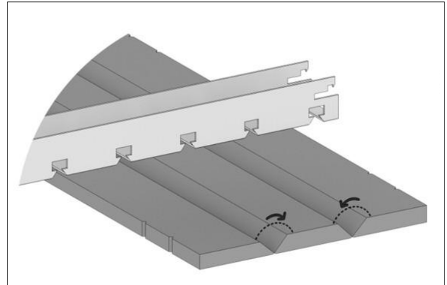
יש לקפל כל למלה לצורת U - 8 למלות לכל אריח
